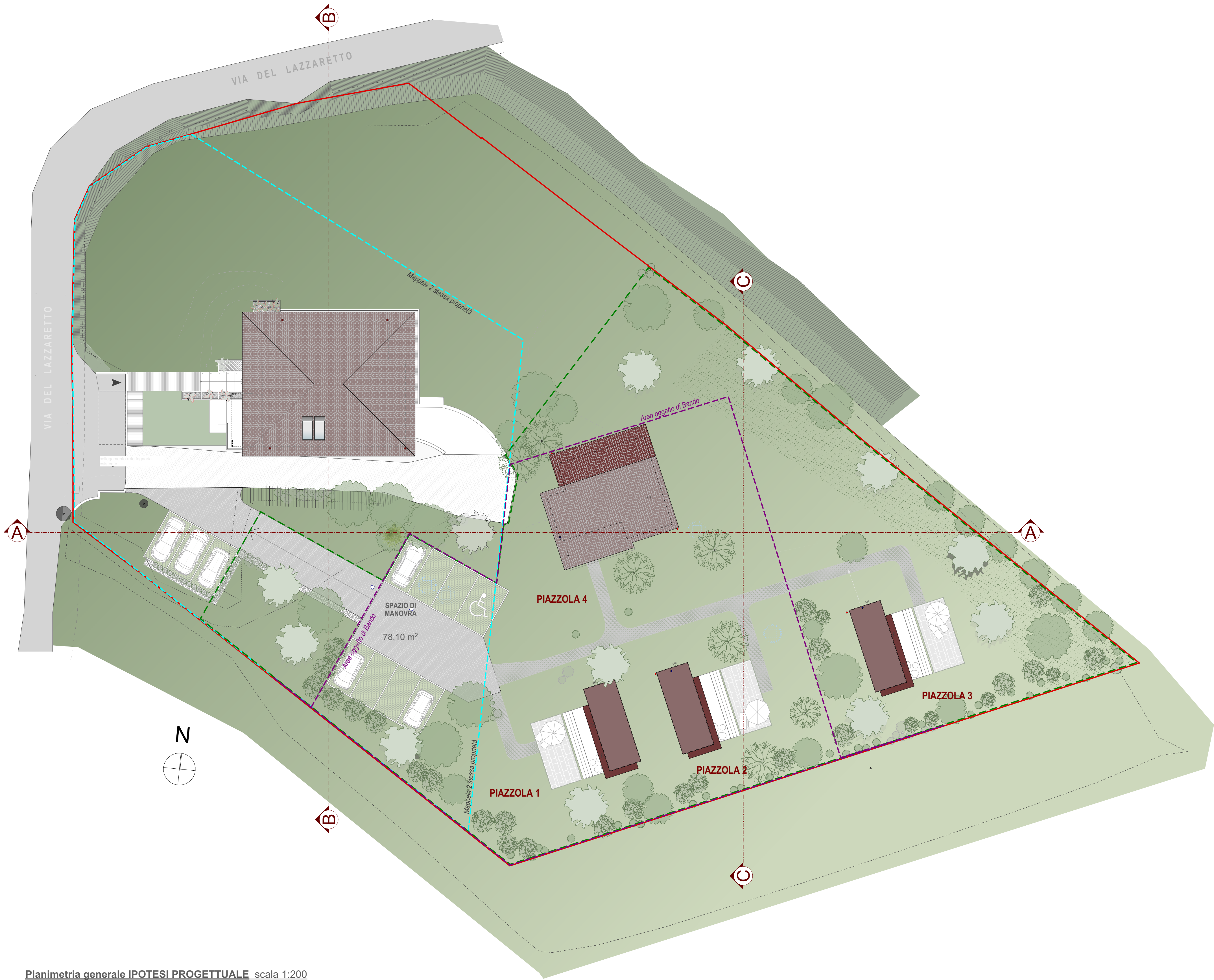
Planimetria generale IPOTESI PROGETTUALE scala 1:200
