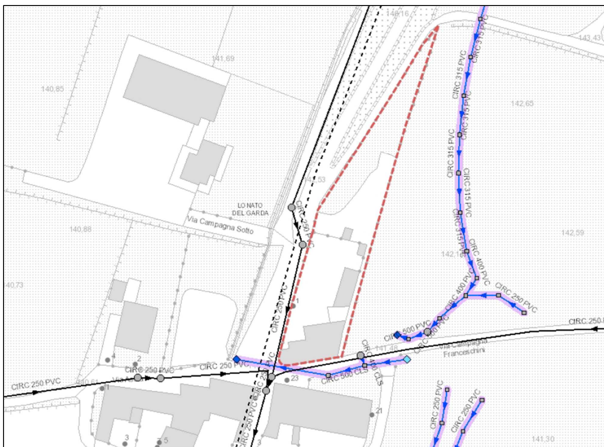
L.01: estratto rete fognaria esistente.
