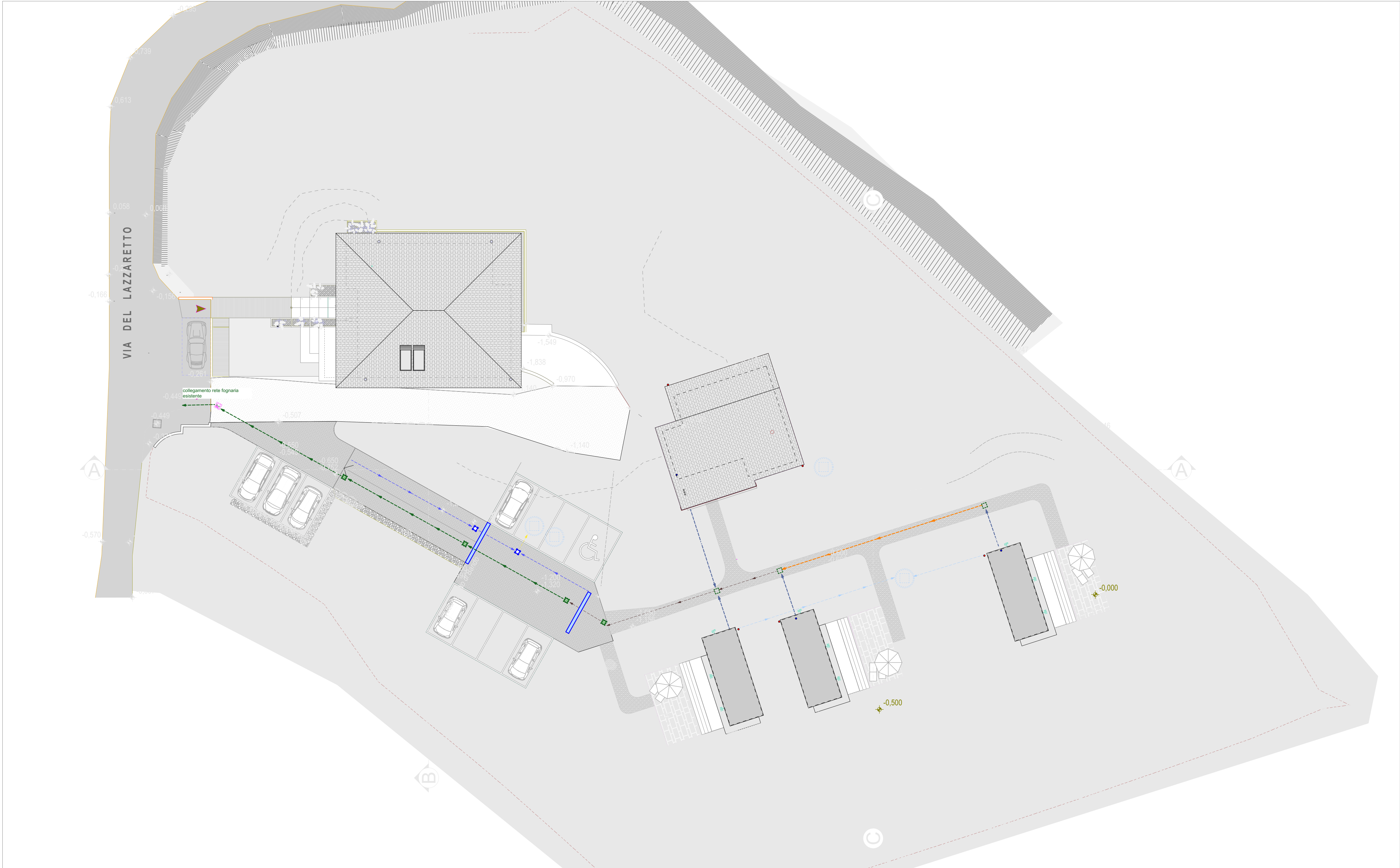
Schema fognario scala 1:200
