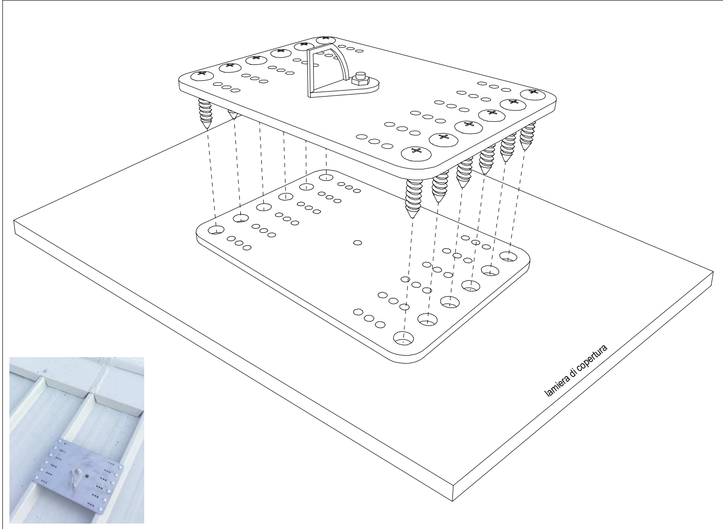
Ancoraggio puntuale permanente UNI 11578 : 2015
