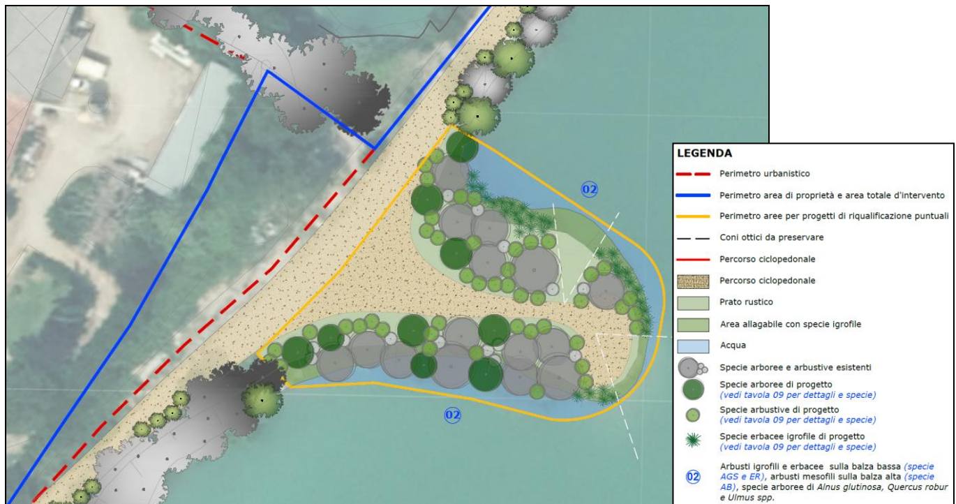
Estratto Tavola 07_ Planimetria di progetto elaborata da StudioZea
