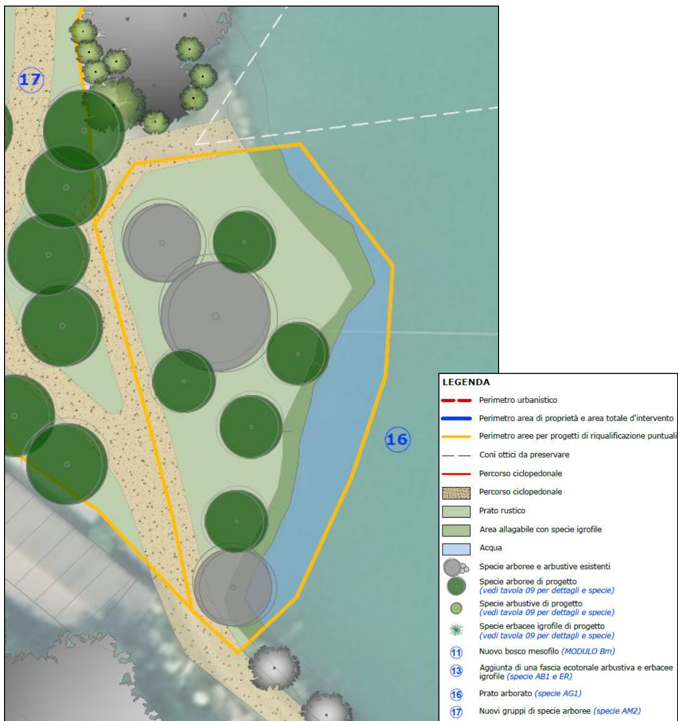
Estratto Tavola 08_ Planimetria di progetto elaborata da StudioZea
