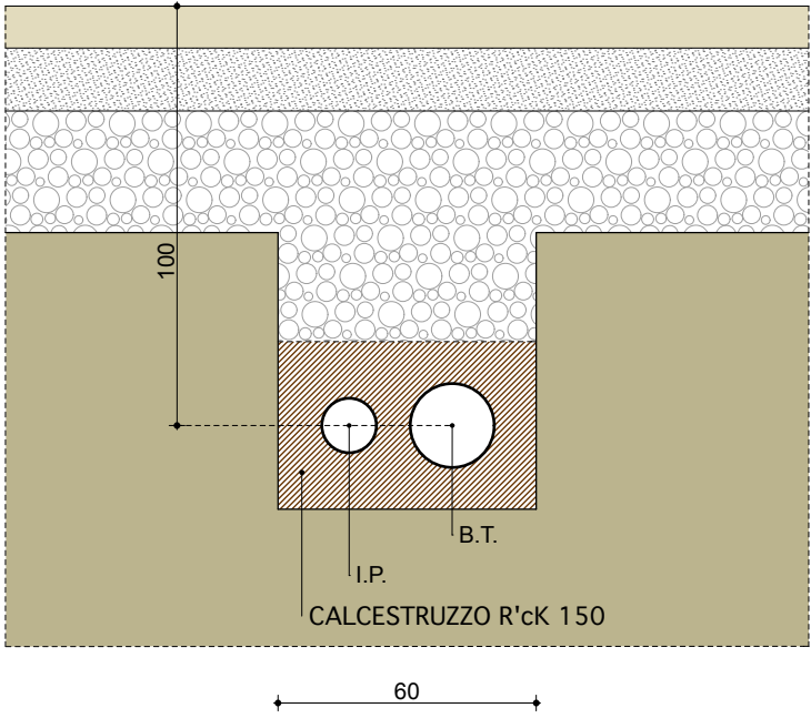
SEZIONE SCAVO E.N.E.L. (B.T.) - ILLUMINAZIONE PUBBLICA
