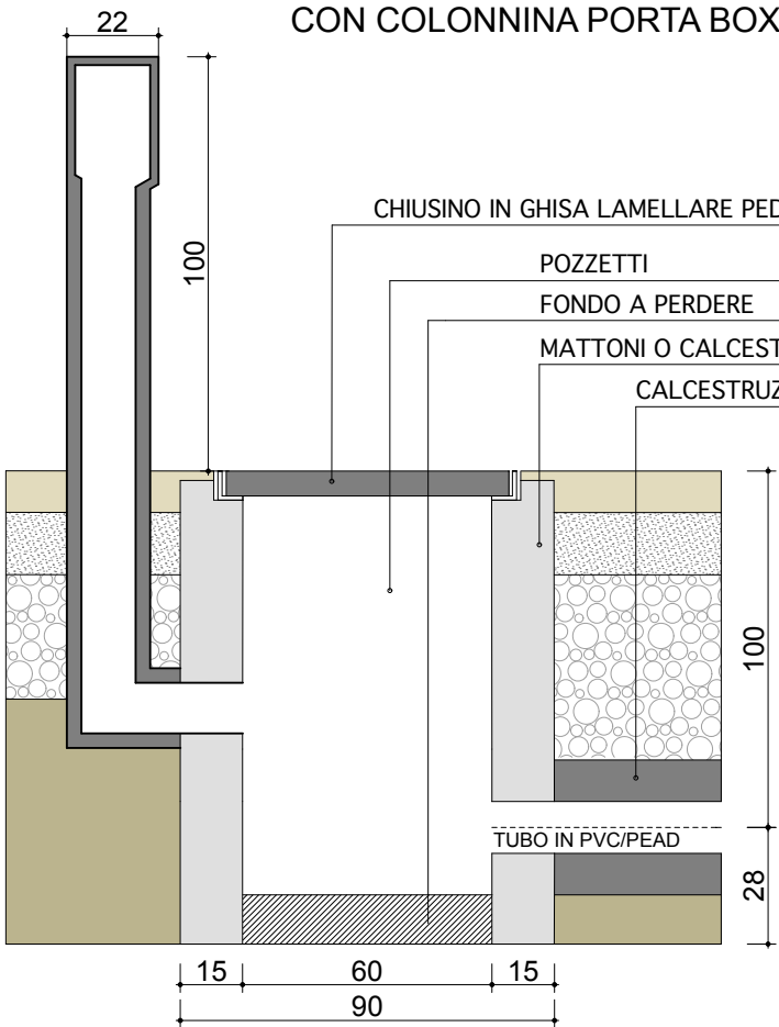
POZZETTO TELECOM cm 60x60 CON COLONNINA PORTA BOX
