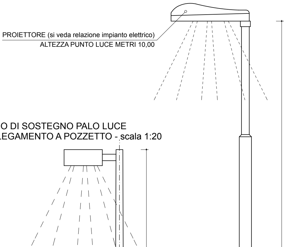
BLOCCO DI SOSTEGNO PALO LUCE E COLLEGAMENTO A POZZETTO
