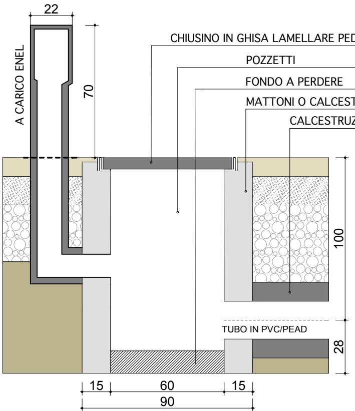
POZZETTO cm 60x60 CON CASSETTA ENEL B.T.
