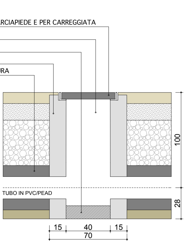
POZZETTO ENEL cm 40x40
