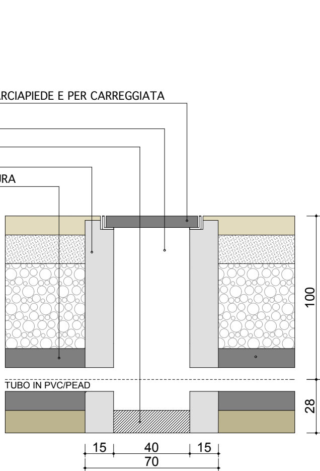
POZZETTO TELECOM cm 40x40
