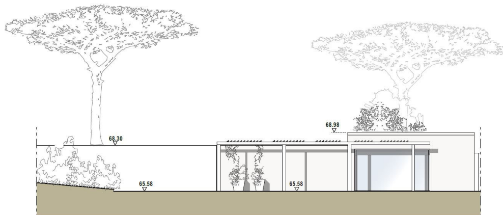
PROSPETTO NORD
