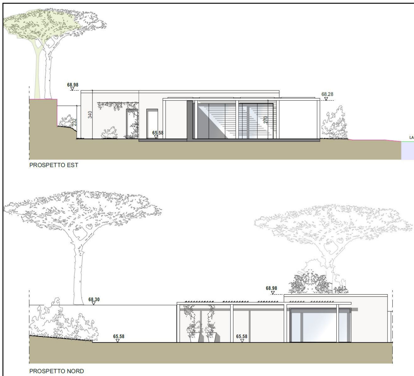
Dettaglio prospetti est - nord
