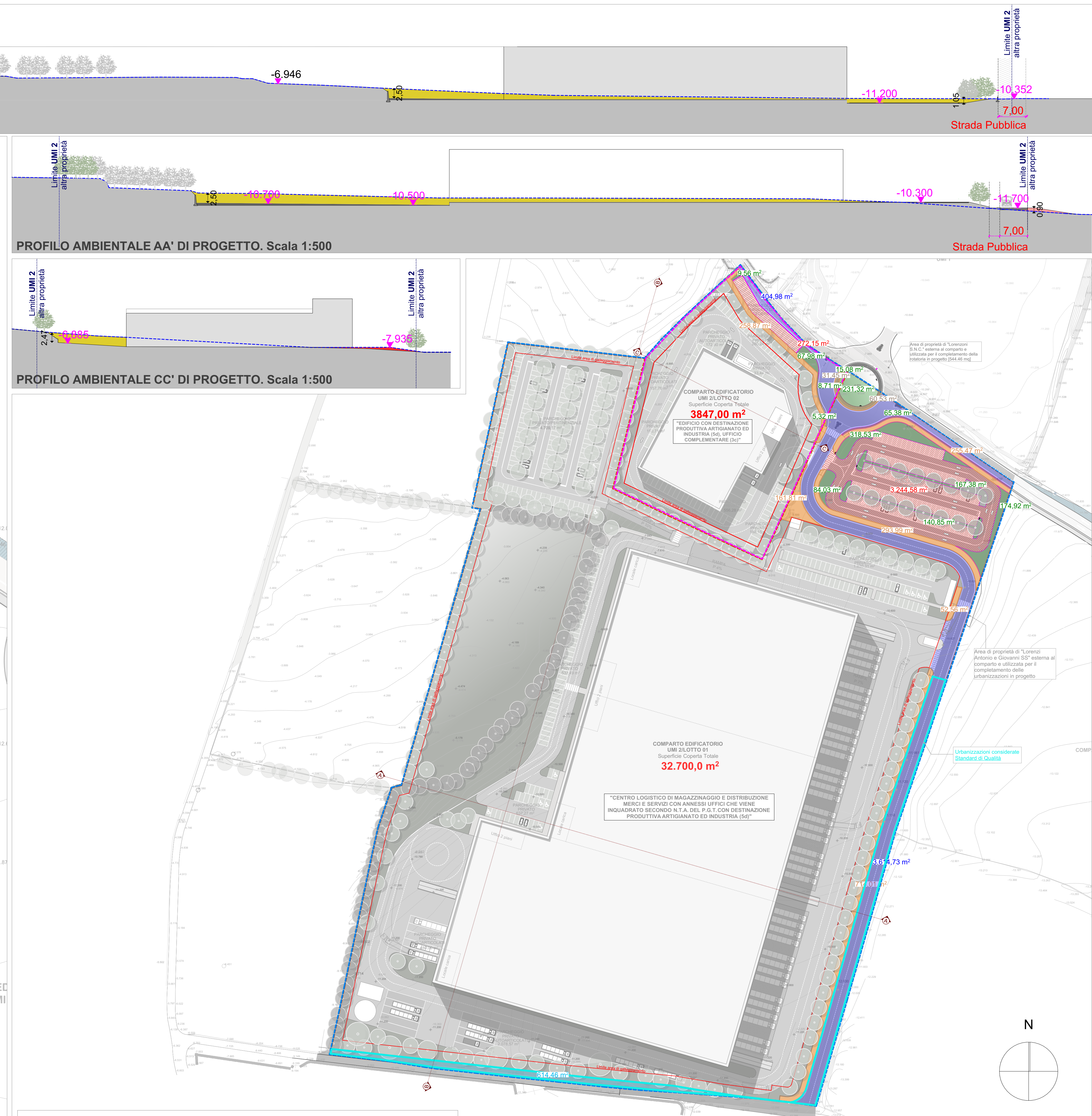
Planimetria Generale di progetto con individuazione aree in cessione Scala 1:1000
