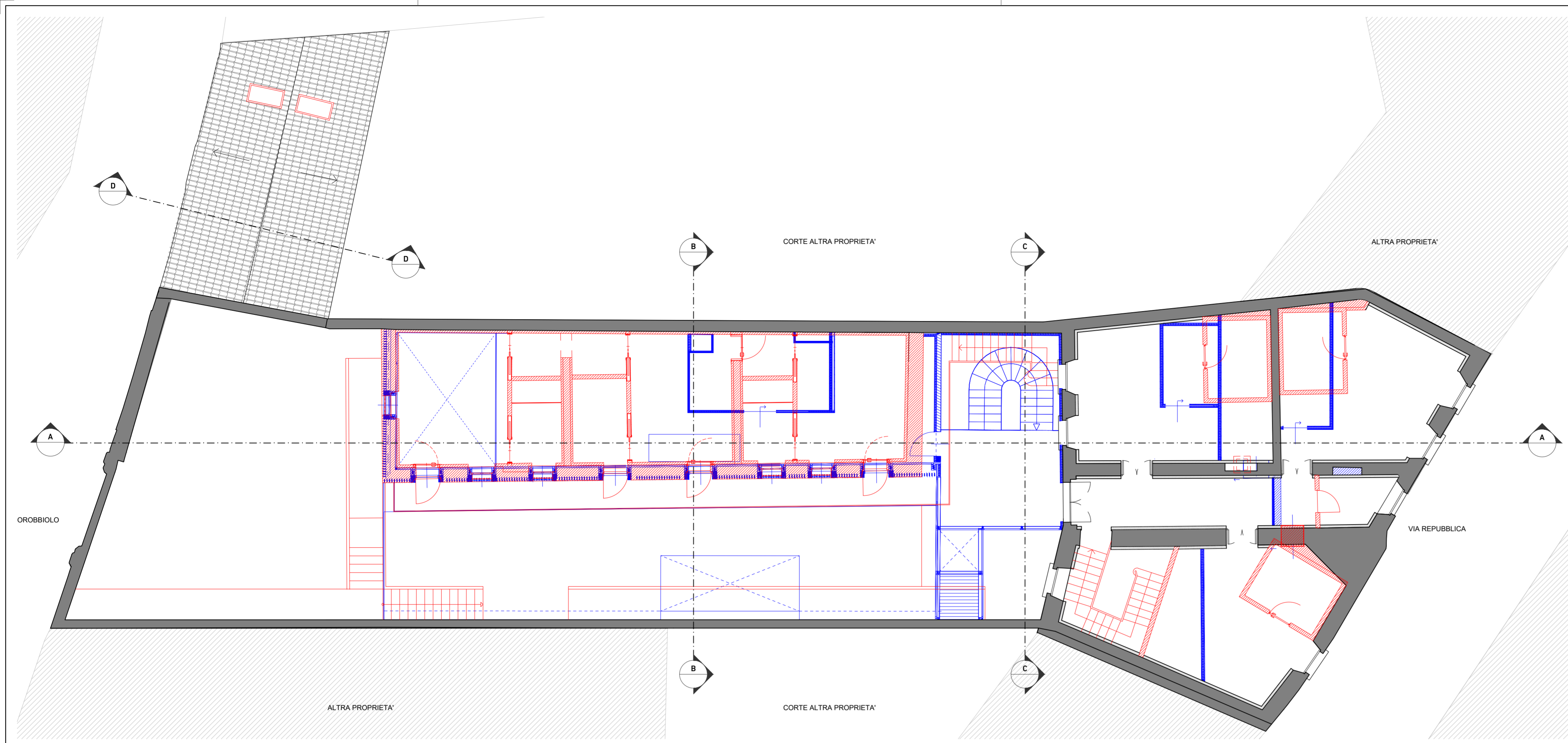
Pianta Piano Primo Stato di Comparazione
