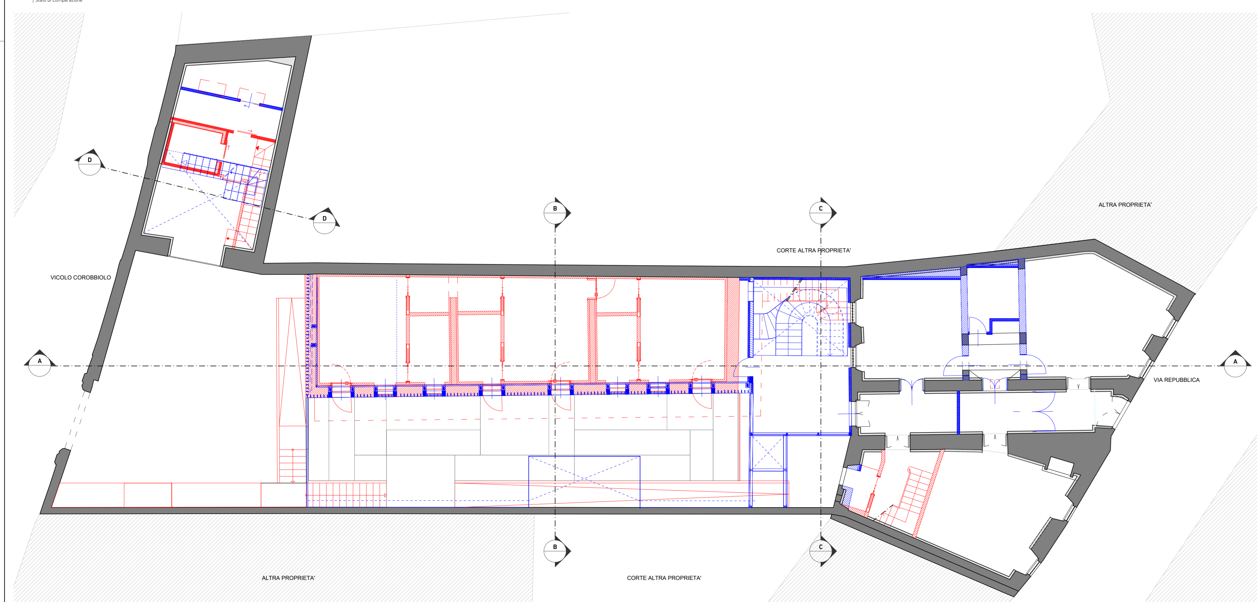
Pianta Piano Terra Stato di Comparazione
