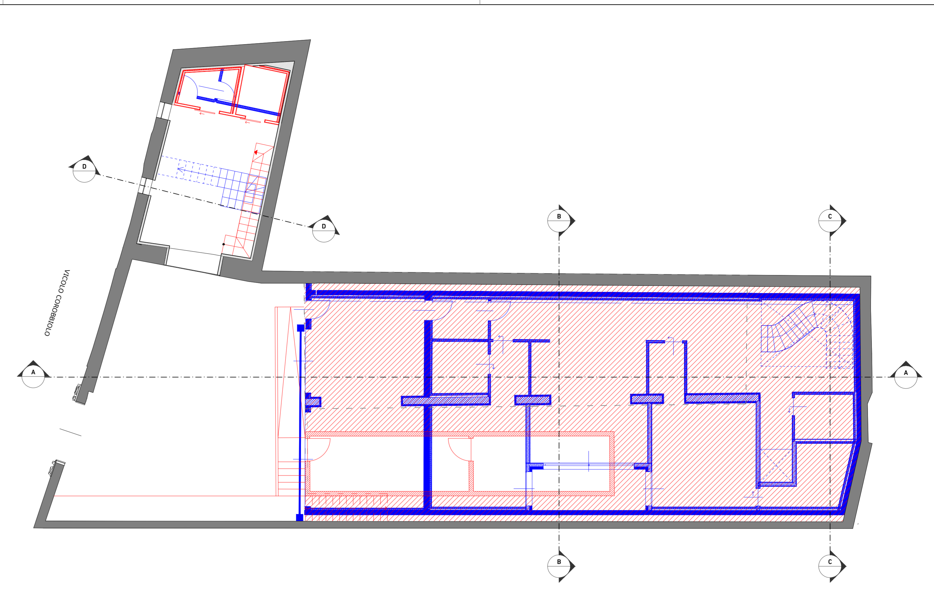
Pianta Piano Interrato Stato di Comparazione
