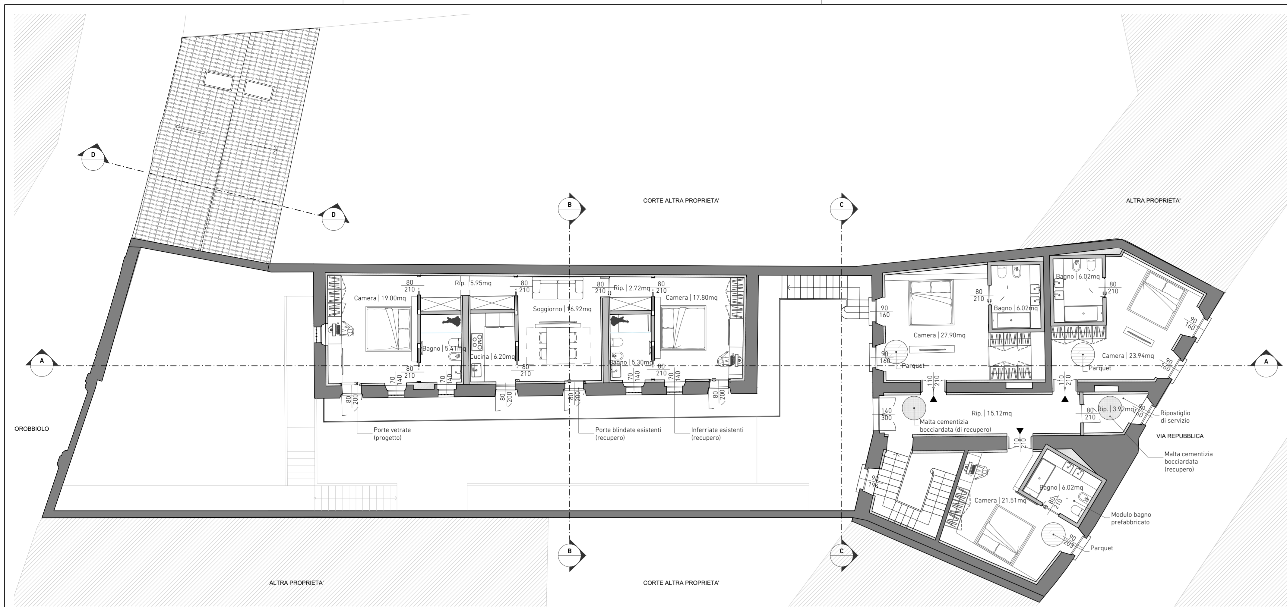
Pianta Piano Primo Stato di Progetto
