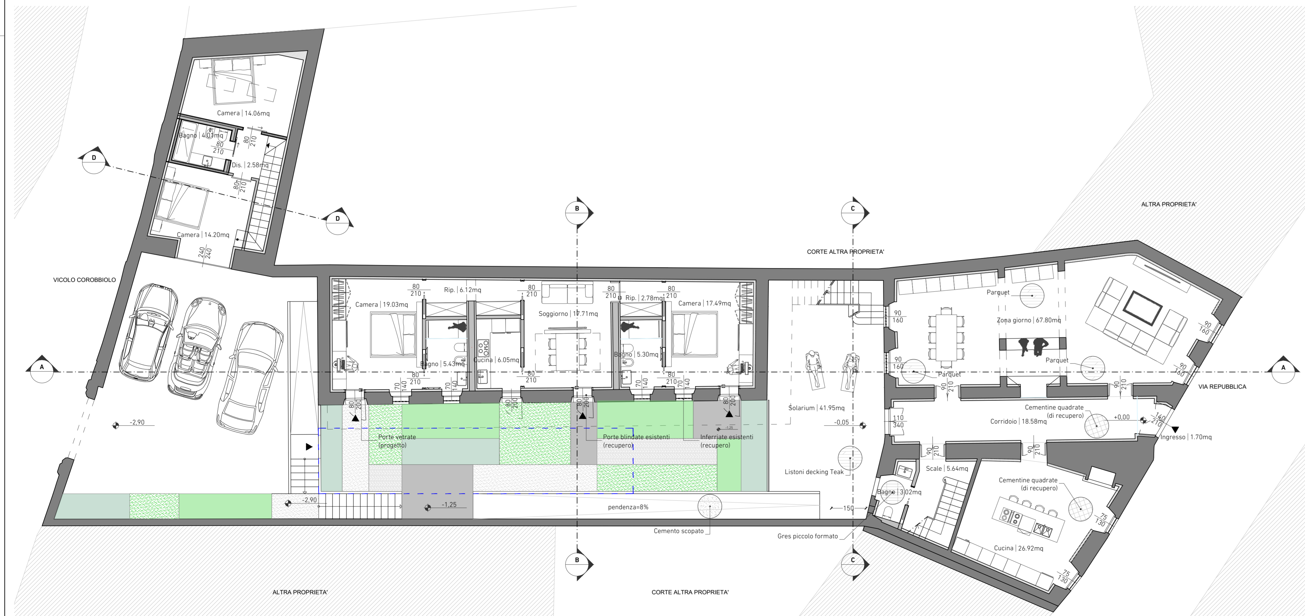
Pianta Piano Terra Stato di Progetto
