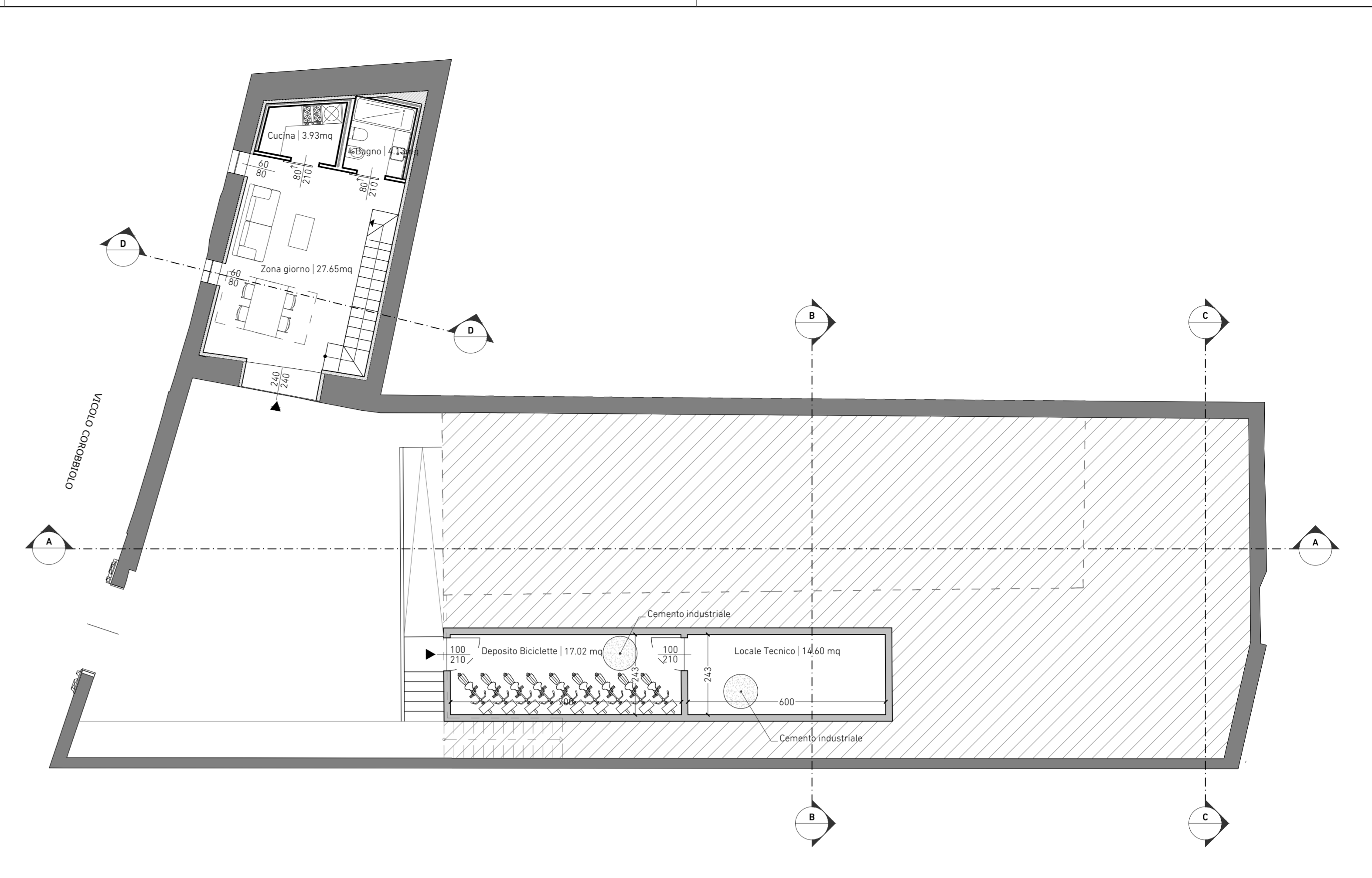
Pianta Piano Interrato Stato di Progetto
